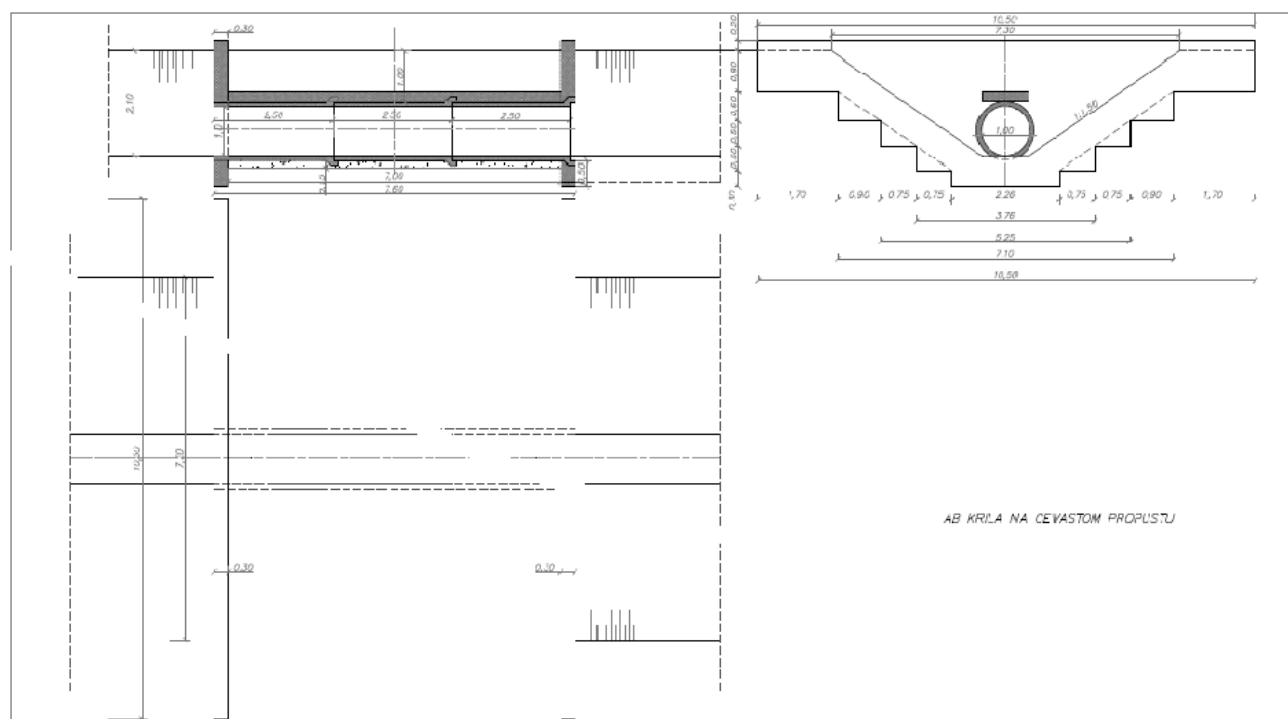
Skica cevastog propusta:
